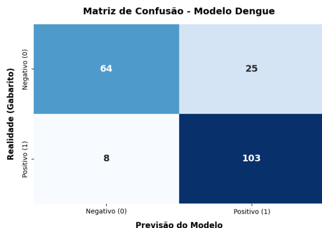
Figura 1. Matriz de Confusão gerada pelas previsões do MLP no conjunto de teste. É notória a taxa de acerto no quadrante de Verdadeiros Positivos (103), em face a um número ínfimo de Falsos Negativos (8).
